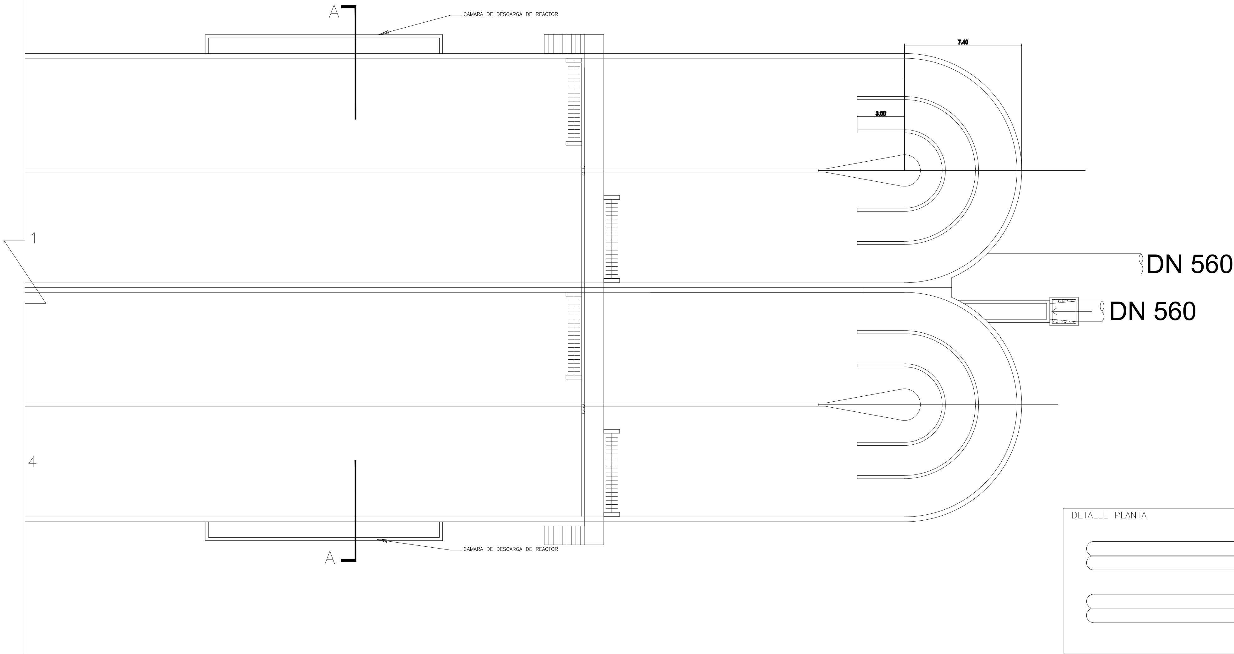
DETALLE PLANTA ESCALA: 1:75
